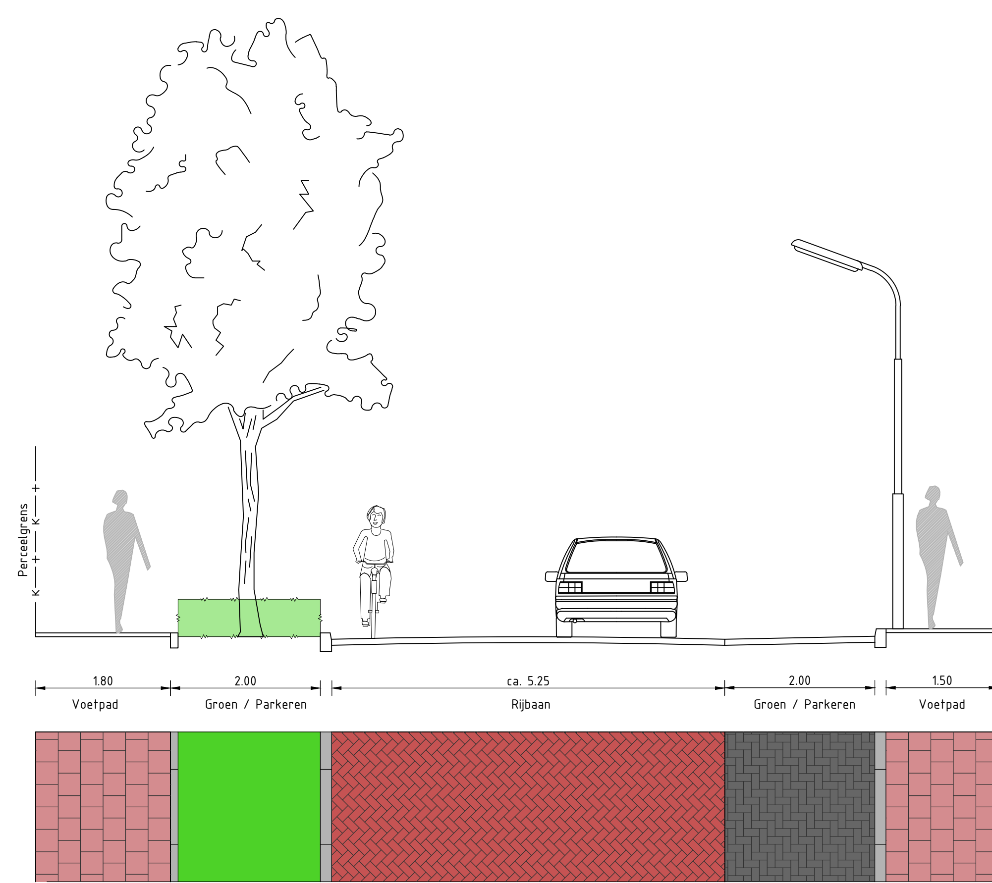
Principeprofiel B Schaal 1 : 50
