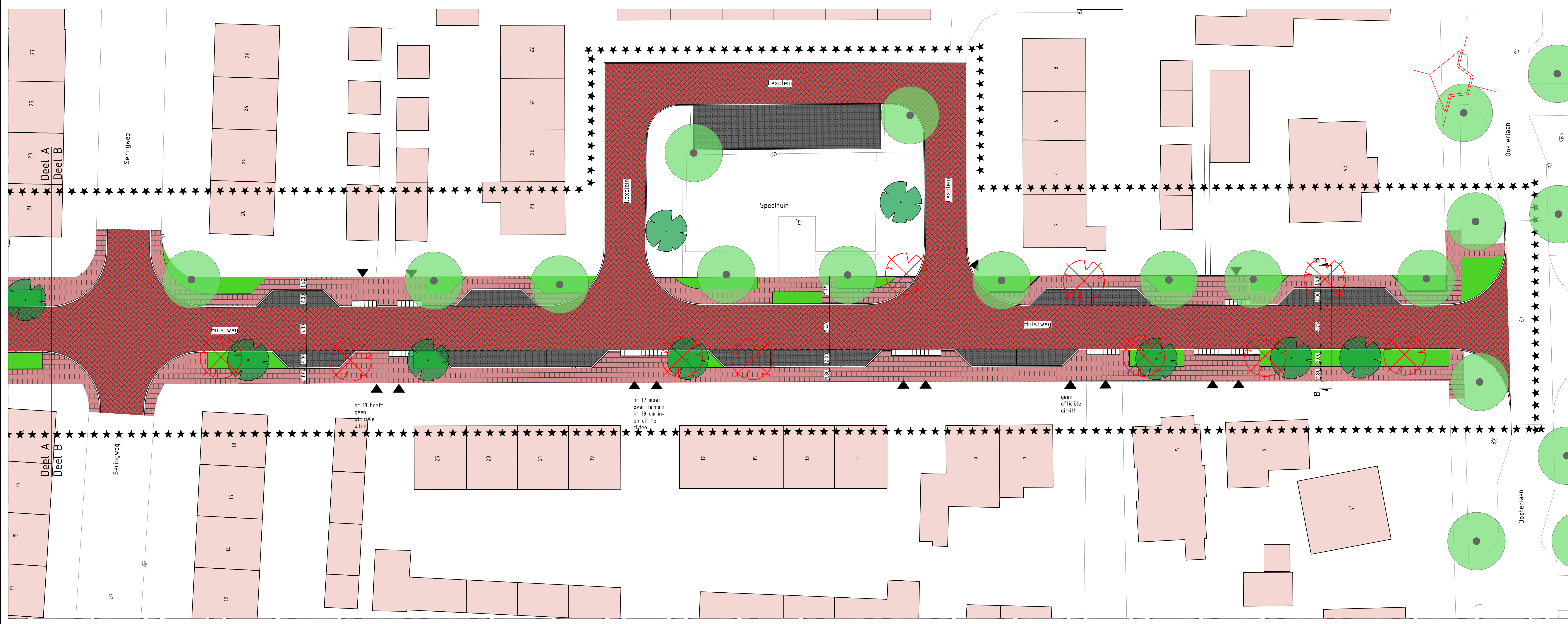
Situatie deel B Schaal 1 : 200
