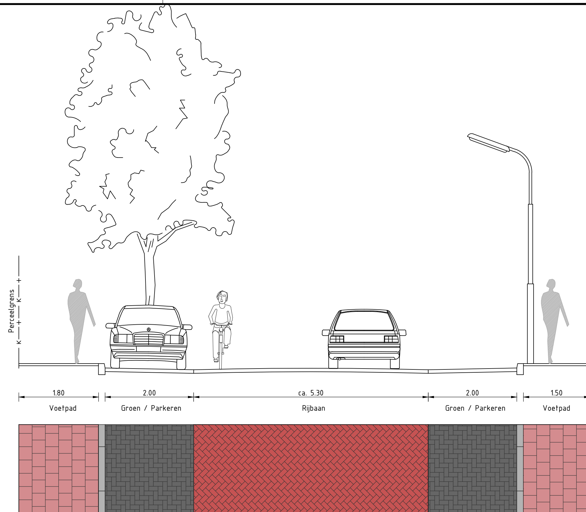
Principeprofiel A Schaal 1 : 50
