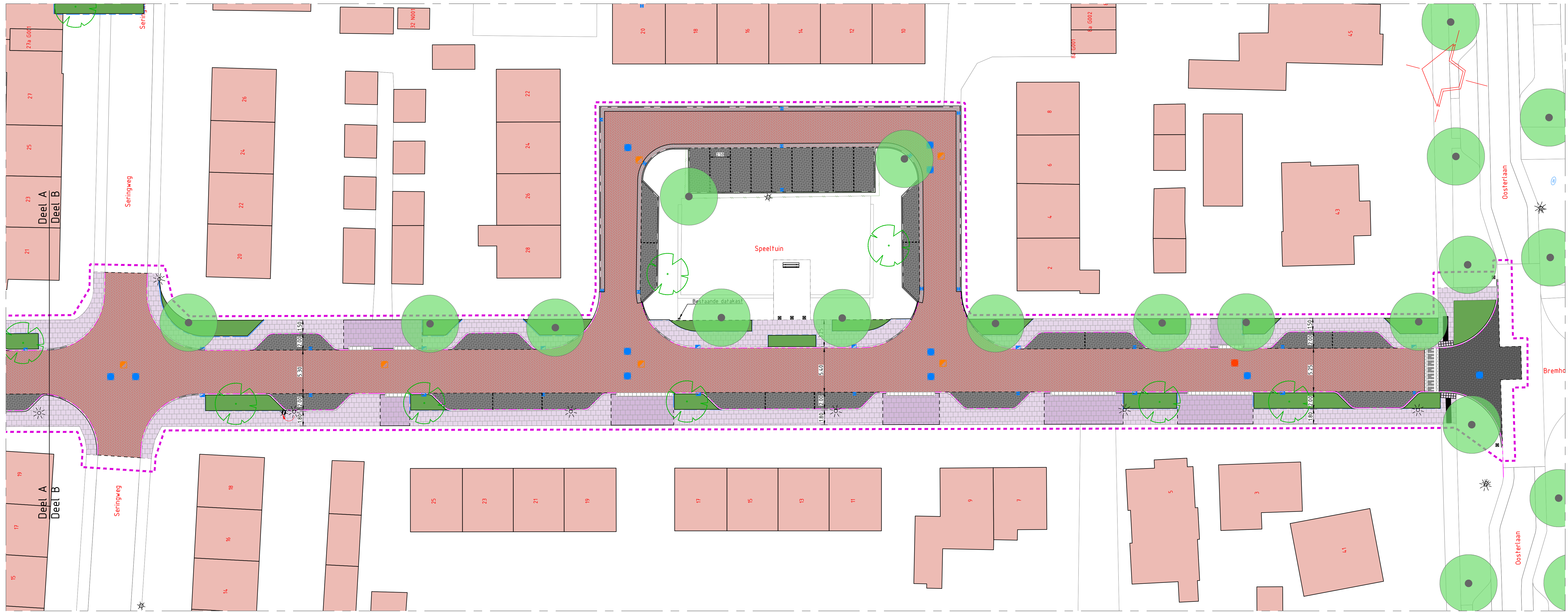
Situatie deel B Schaal 1 : 200
